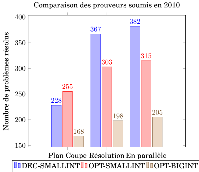
FIGURE 4.10 – Performance des différents prouveurs pseudo-bouliens de Sat4j 2.2.1 dans les conditions de PB 2010 : nombre de benchmarks résolus dans chaque catégorie parmi respectivement 452, 699 et 532 benchmarks.
