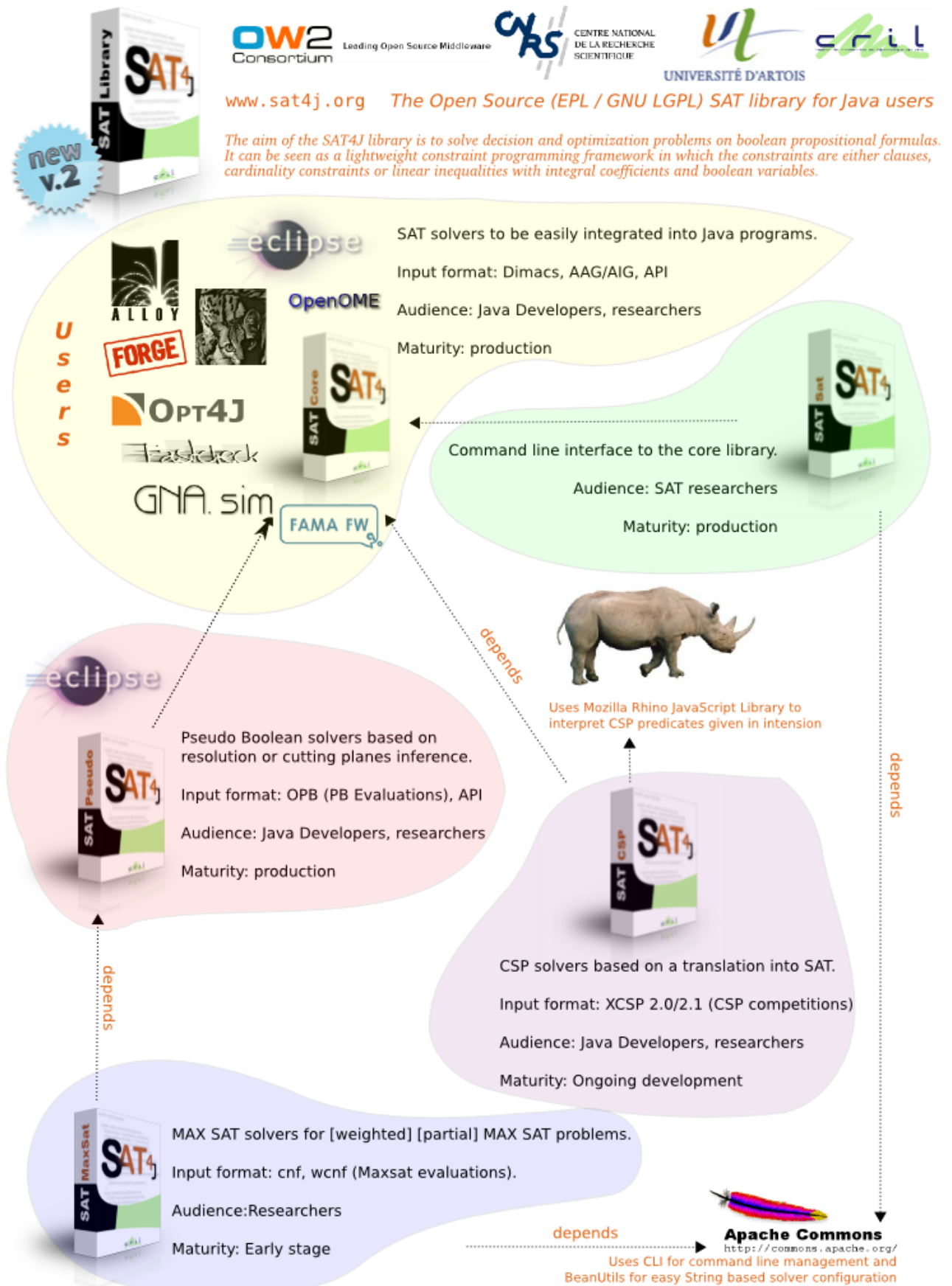
FIGURE 4.1 – Architecture de Sat4j depuis la version 2.0
